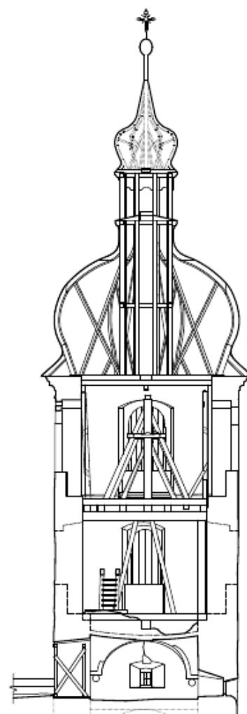
Příčný řez zvonice. UJEP, Terra Sacra Incognita
